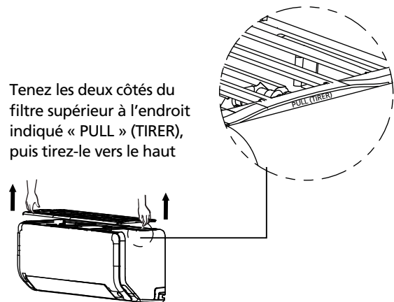
Fig.17 –Maintenir et tirer le filtre
