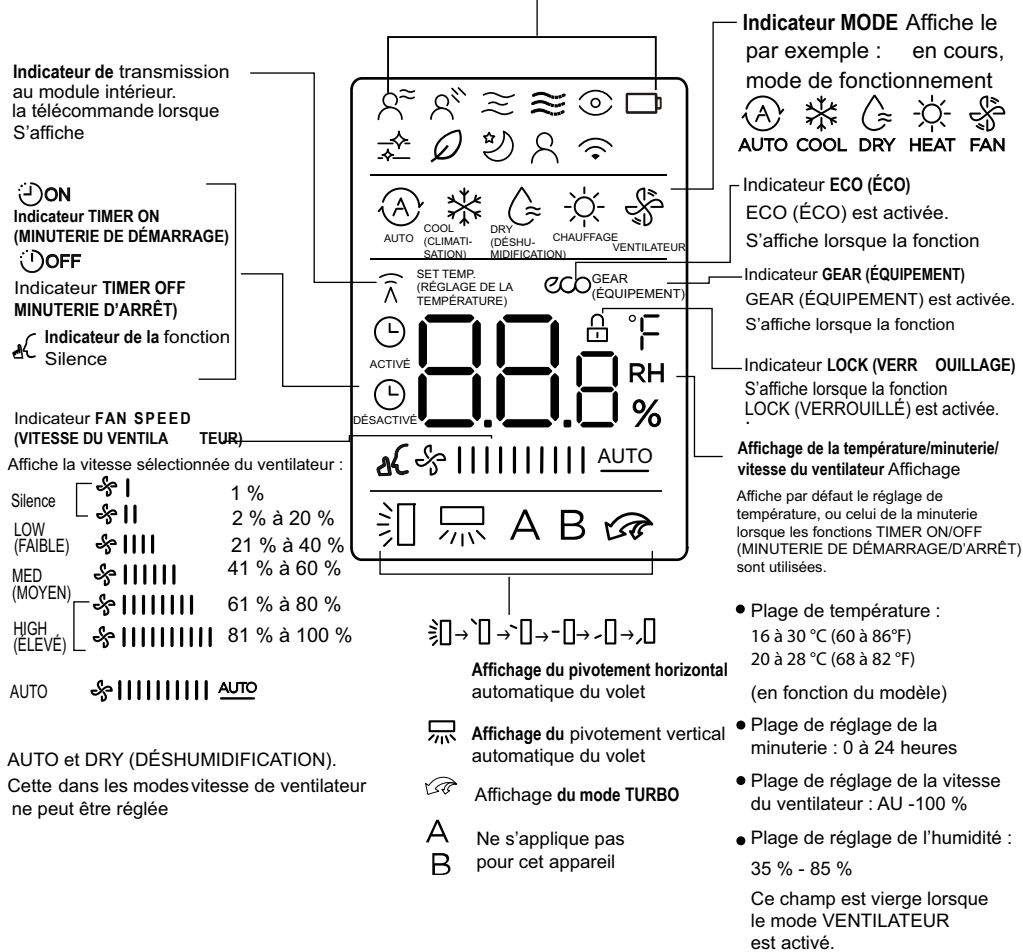
Fig.3 –Indicateurs de la télécommande sans fil
